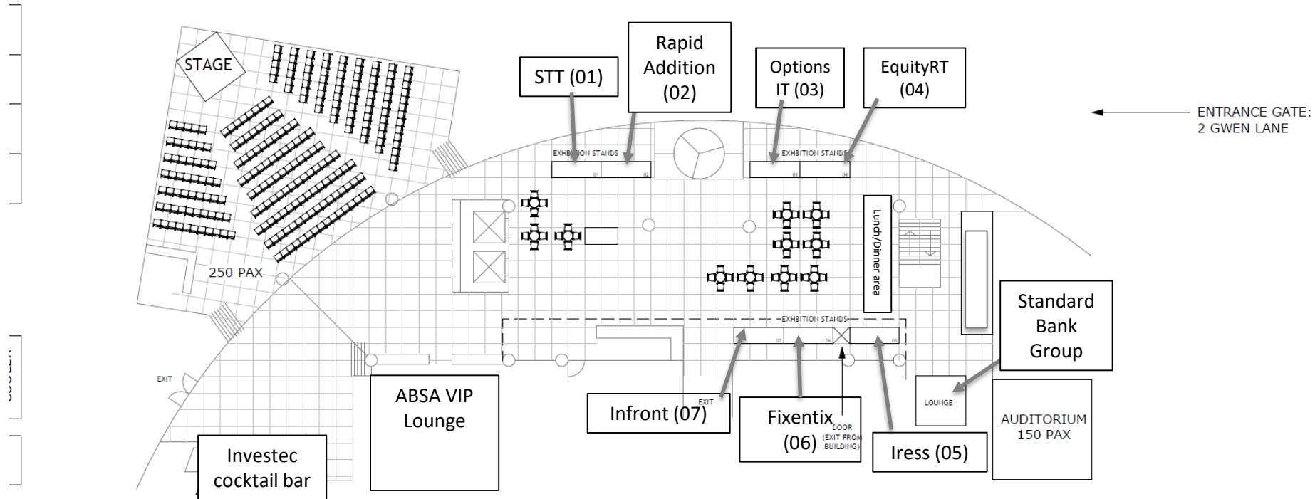
STAND LAYOUT 1 : 220
